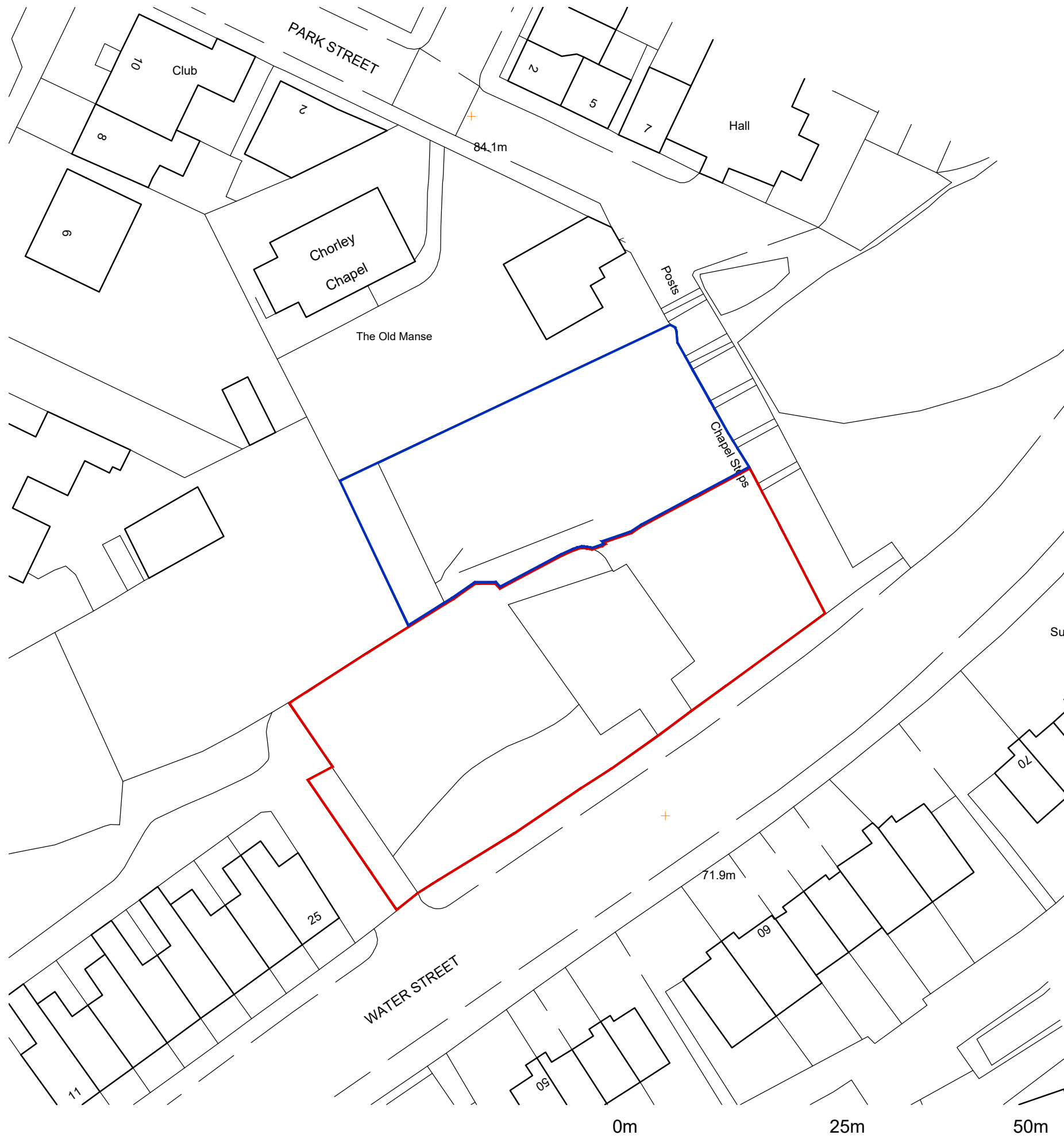
Site Layout 1:500
