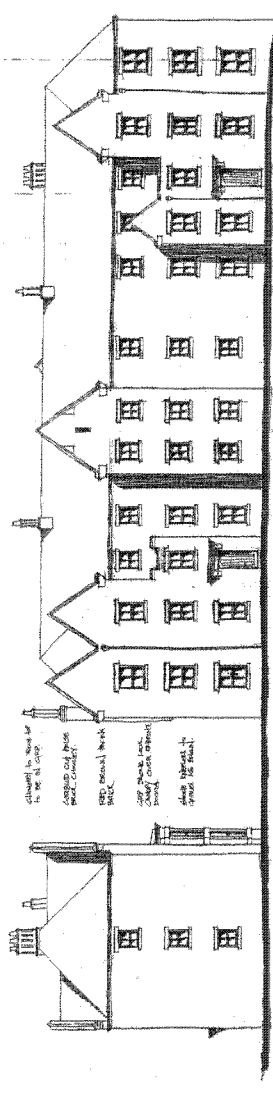
Elevation 3
