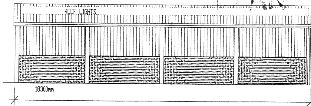
ELEVATION A
